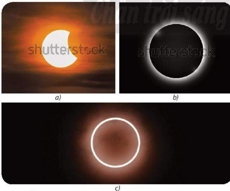
▲ Hình 6.1. a) Nhật thực một phần; b) Nhật thực toàn phần; c) Nhật thực hình khuyên
