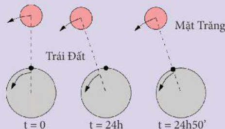
▲ Hình 6.17. Ảnh hưởng từ sự quay của Mặt Trăng xung quanh Trái Đất và sự tự quay quanh trục của Trái Đất đến hiện tượng thủy triều
