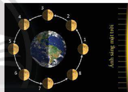
▲ Hình 5.16. Vị trí các pha của Mặt Trăng nhìn từ phần tối của Trái Đất
