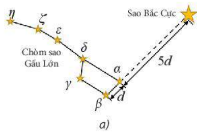
▲ Hình 4.6. Xác định sao Bắc Cực từ chòm sao: a) Gấu Lớn; b) Thiên Hậu
