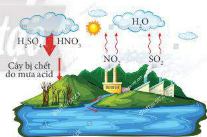
▲ Hình 10.6. Quy trình tạo thành mưa acid
