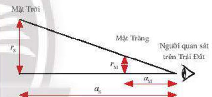
Hình 6.7. Minh họa sự đồng dạng giữa Mặt Trăng và Mặt Trời đối với người quan sát trên Trái Đất
