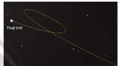
▲ Hình 5.8. Chuyển động nhìn thấy của Thủy tinh (Nguồn: Stellarium)
