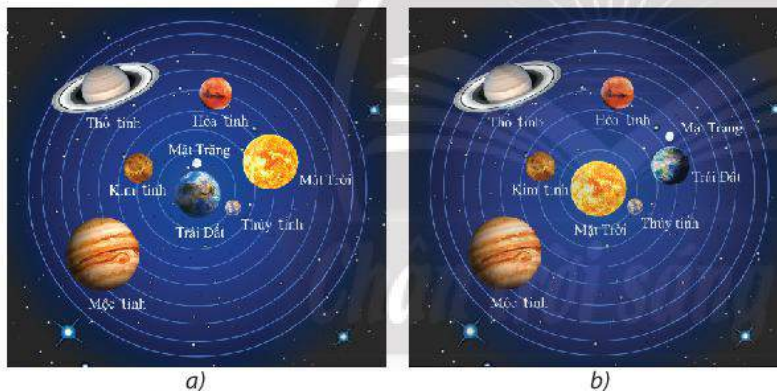
▲ Hình 5.11. Mô hình: a) hệ địa tâm của Ptolemy; b) hệ nhật tâm của Copernicus
