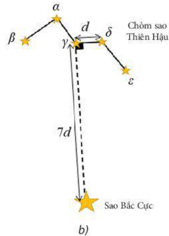
▲ Hình 4.6. Xác định sao Bắc Cực từ chòm sao: a) Gấu Lớn; b) Thiên Hậu
