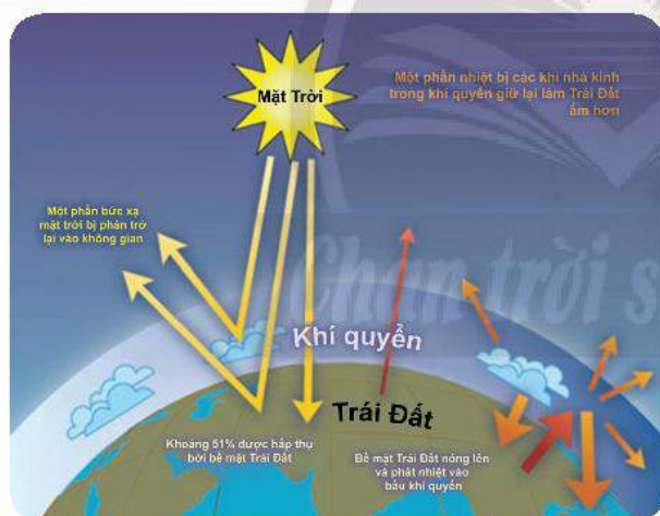
Hình 10.4. Hiệu ứng nhà kính làm Trái Đất nóng lên
