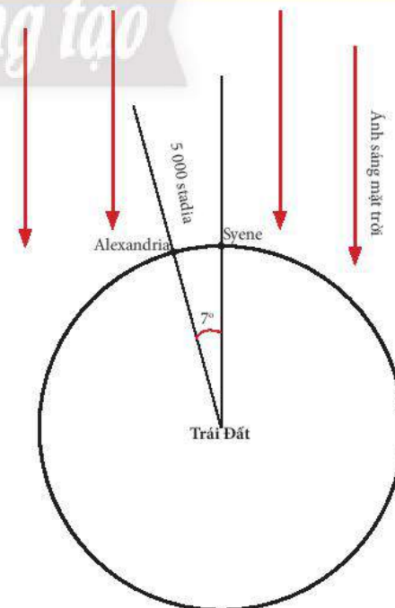
▲ Hình 5.9. Mô hình tính chu vi Trái Đất
