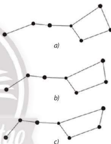
Hình 4.2. Minh họa vị trí tương đối giữa các ngôi sao trong chòm sao Gấu Lớn vào thời điểm:
