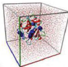
▲ Hình 3.18. Mô phỏng MD để nghiên cứu DNA
