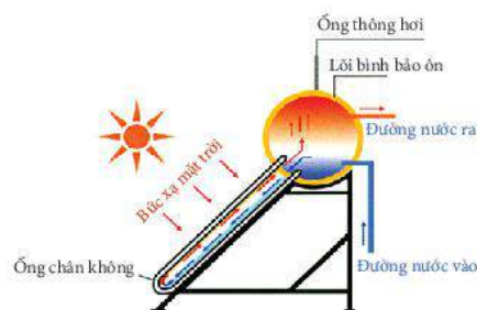
▲ Hình 8.8. Nguyên lý hoạt động của máy nước nóng năng lượng mặt trời
