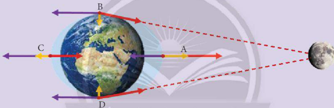
▲ Hình 6.16. Minh họa lực tương tác giữa Mặt Trăng và các khối nước trên bề mặt Trái Đất
