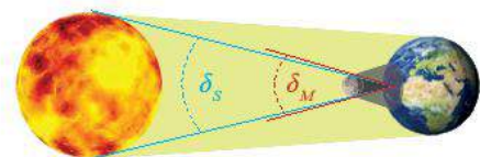
a) Nhật thực toàn phần
