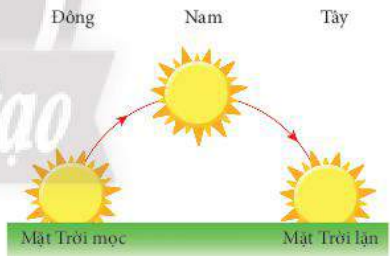
▲ Hình 5.1. Chuyển động nhìn thấy của Mặt Trời ở Bắc bán cầu
