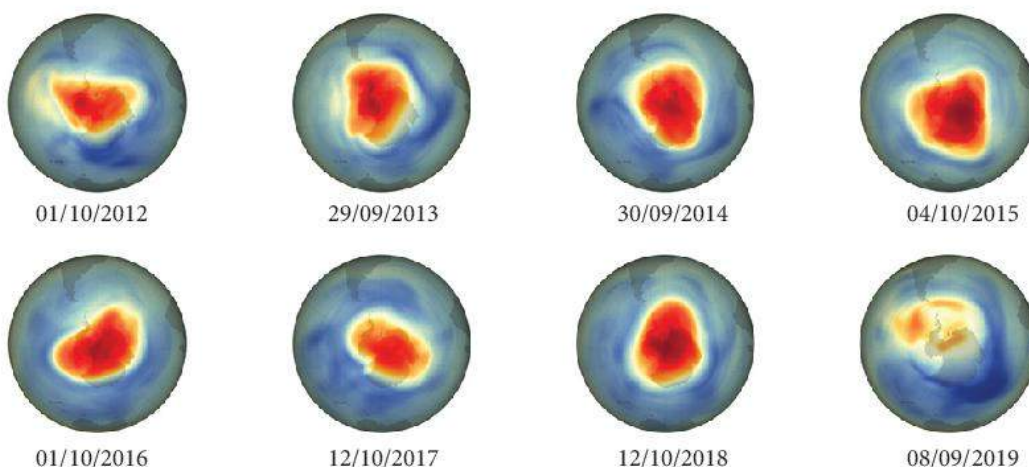
▲ Hình 10.15. Hình dạng và kích thước lỗ thủng ozone từ năm 2012 đến năm 2019
