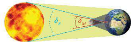
b) Nhật thực hình khuyên
