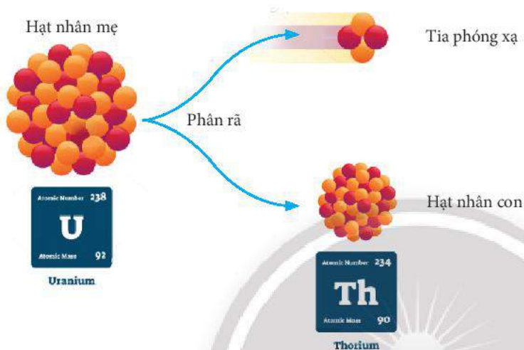
▲ Hình 10.7. Quá trình phân rã phóng xạ
