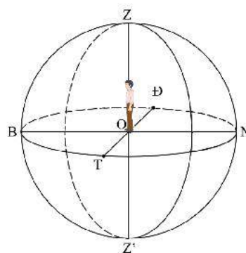
Hình 4.1. Minh họa thiên cầu
