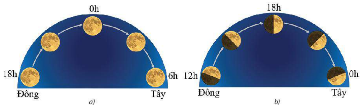
▲ Hình 5.4. Hình ảnh quan sát tại mặt đất về đường đi của Mặt Trăng trên bầu trời vào: a) ngày rằm; b) ngày 8 âm lịch hằng tháng
