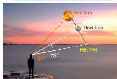
▲ Hình 5.6. Li giác cực đại của Kim tinh và Thủy tinh nhìn từ Trái Đất
