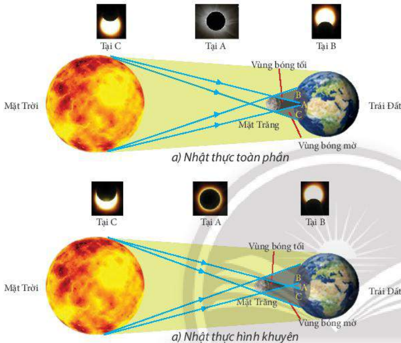
▲ Hình 6.4. Hình ảnh nhật thực quan sát được tại các vị trí khác nhau trên Trái Đất trong hai trường hợp nhật thực toàn phần và nhật thực hình khuyên
