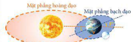
▲ Hình 5.13. Tương quan giữa mặt phẳng hoàng đạo và bạch đạo tại một số thời điểm trong năm
