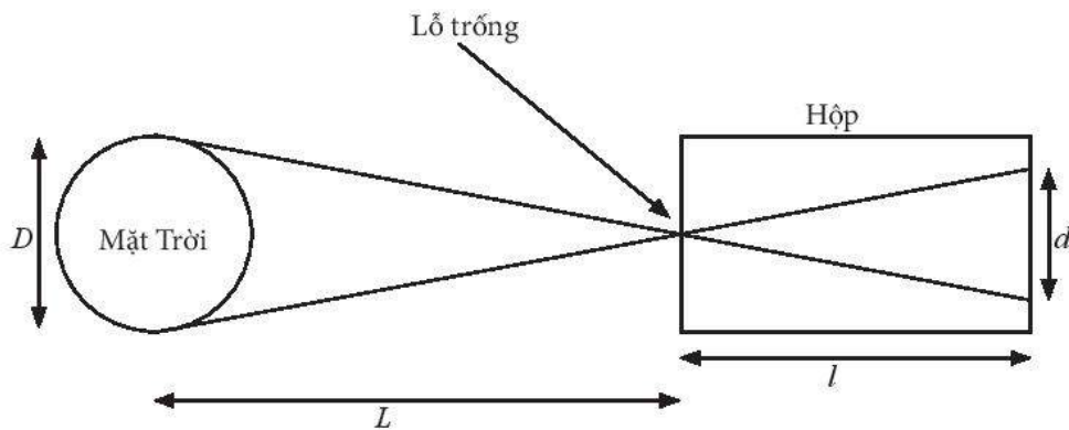
▲ Hình 6P.3. Mô hình đơn giản Aristarchus sử dụng đo đường kính của Mặt Trời
