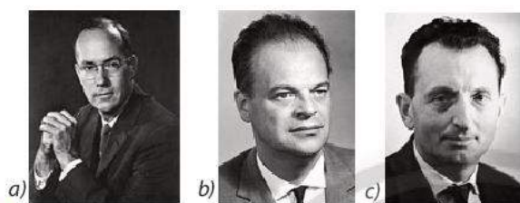
▲ Hình 2.7. Các nhà vật lý đặt nền móng lý thuyết cho sự phát triển của laser: a) Charles H. Townes (1915 – 2015); b) Nikolay Basov (1922 – 2001); c) Alexander Prokhorov (1916 – 2002)
