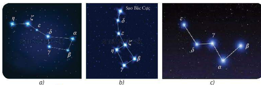
Hình 4.4. Ba chòm sao: a) Gấu Lớn; b) Gấu Nhỏ; c) Thiên Hậu
