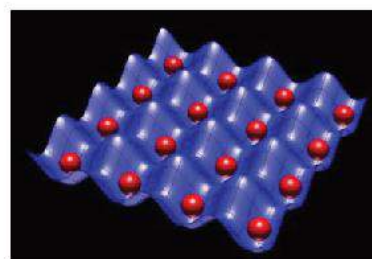
▲ Hình 2.17. Mạng quang học
