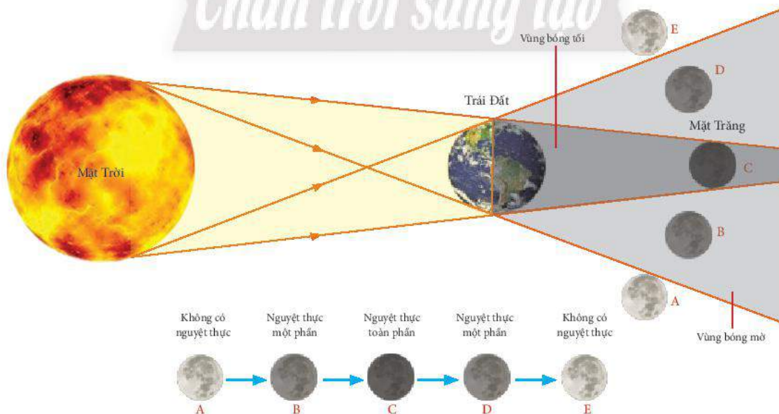
▲ Hình 6.9. Quá trình diễn ra hiện tượng nguyệt thực
