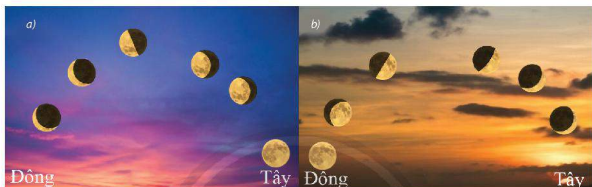
▲ Hình 5.5. Vị trí của Mặt Trăng vào 6 ngày khác nhau trong một Tuần Trăng tại hai thời điểm: a) bình minh; b) hoàng hôn
