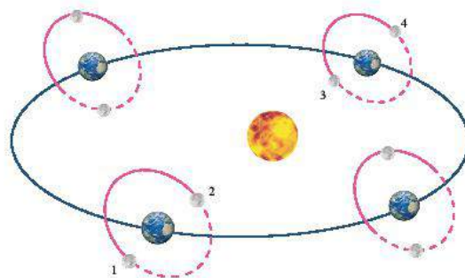
▲ Hình 6.11. Minh họa điều kiện diễn ra nhật thực và nguyệt thực. Hiện tượng nhật thực diễn ra khi Mặt Trăng ở vị trí 2 và 3, hiện tượng nguyệt thực diễn ra khi Mặt Trăng ở vị trí 1 và 4
