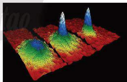
▲ Hình 2.16. Hình ảnh mô tả phân bố vận tốc của các nguyên tử khí ^{87}\text{Rb} trong thí nghiệm xác nhận sự tồn tại của BEC
