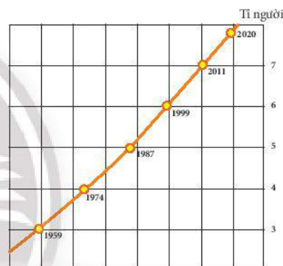
▲ Hình 7.3. Biểu đồ gia tăng dân số thế giới từ năm 1959 cho đến nay theo đơn vị tỉ người (Nguồn số liệu: danso.org)
