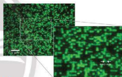
▲ Hình 2.18. Ảnh chụp các nguyên tử bị giam trong mạng quang học
