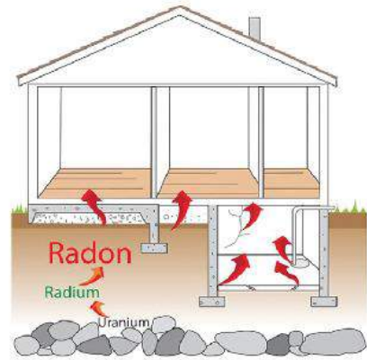
▲ Hình 10.10. Cách thức khí radon-86 đi vào các công trình nhà ở
