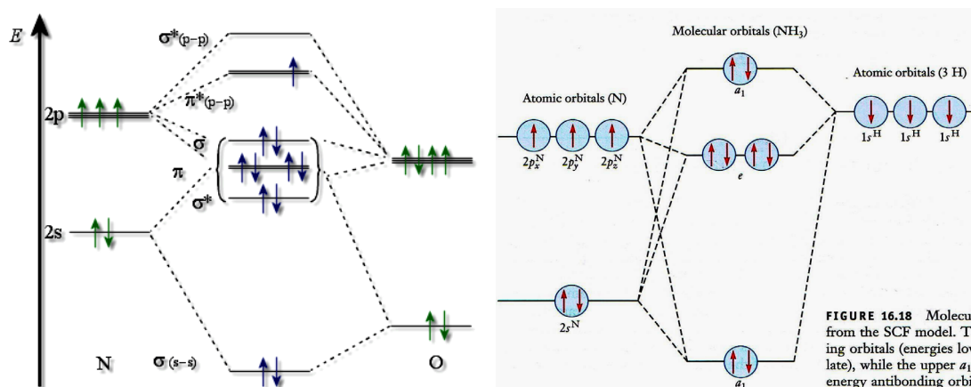
Hình 4.9. MO một số hợp chất khác
