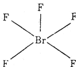
Br lai hóa \text{sp}^3\text{d}^2 \text{BrF}_5 : dạng tháp vuông
