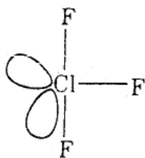
Cl lai hóa \text{sp}^3\text{d} \text{ClF}_3 : dạng chữ T
