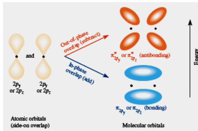
Hình 4.6. Tổ hợp các AO tạo MO
