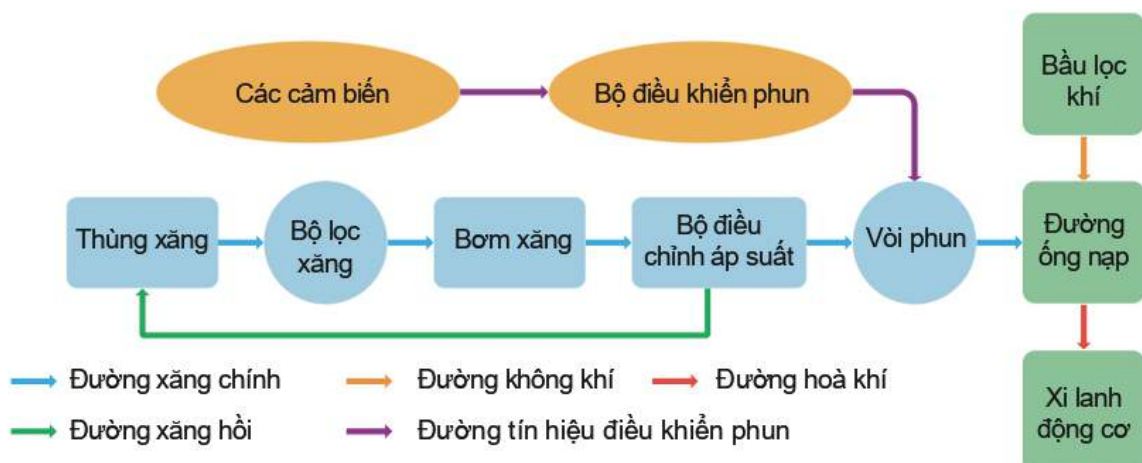
Hình 20.6. Sơ đồ hệ thống phun xăng
