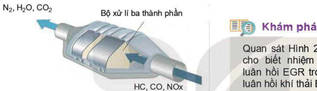
Hình 20.12. Cấu tạo của bộ xử lí ba thành phần
