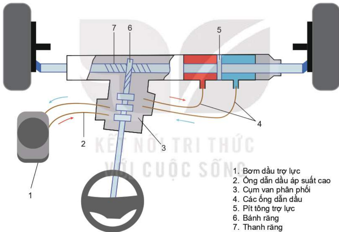
Hình 24.5. Hệ thống trợ lực lái
