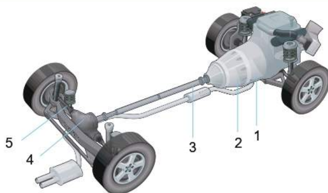
Hình 22.2. Hệ thống truyền lực ô tô
