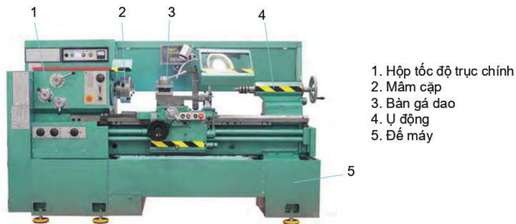
Hình 8.7. Máy tiện vạn năng
