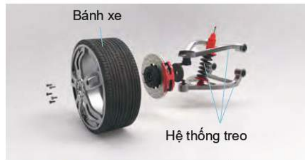
Hình 21.5. Bánh xe và hệ thống treo
