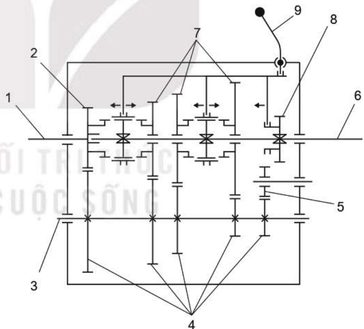
Hình 22.4. Hộp số thường ba trục
