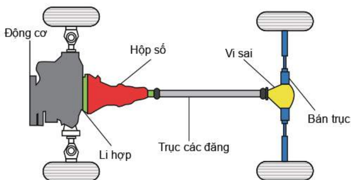
Hình 21.4. Hệ thống truyền lực trên ô tô
