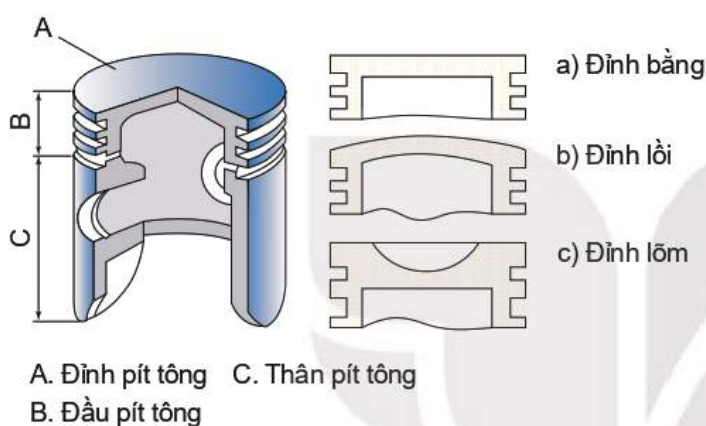
Hình 19.3. Cấu tạo
