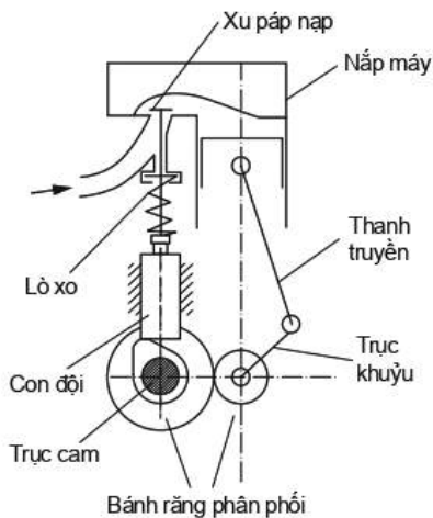
Hình 19.7. Sơ đồ cấu tạo của cơ cấu phôi khí dùng xu páp đặt
