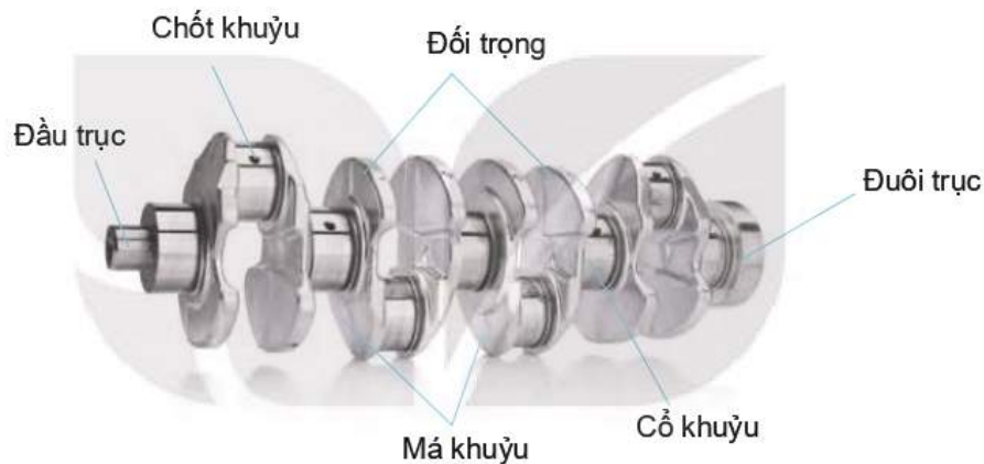
Hình 19.5. Cấu tạo trục khuỷu
