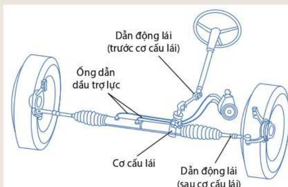
Hình 24.2. Cấu tạo chung của hệ thống lái
