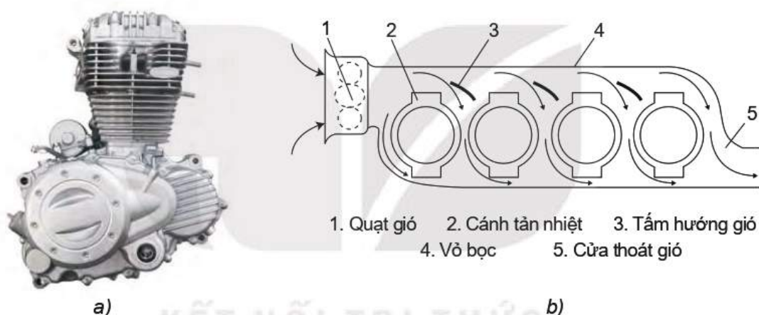
Hình 20.4. Hệ thống làm mát bằng không khí
