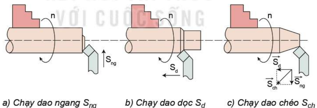
Hình 8.8. Các chuyển động khi tiện
