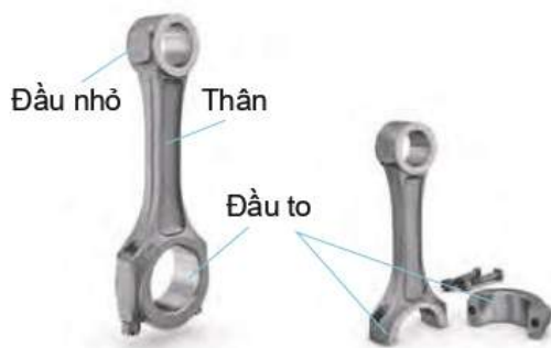
Hình 19.4. Cấu tạo thanh truyền
