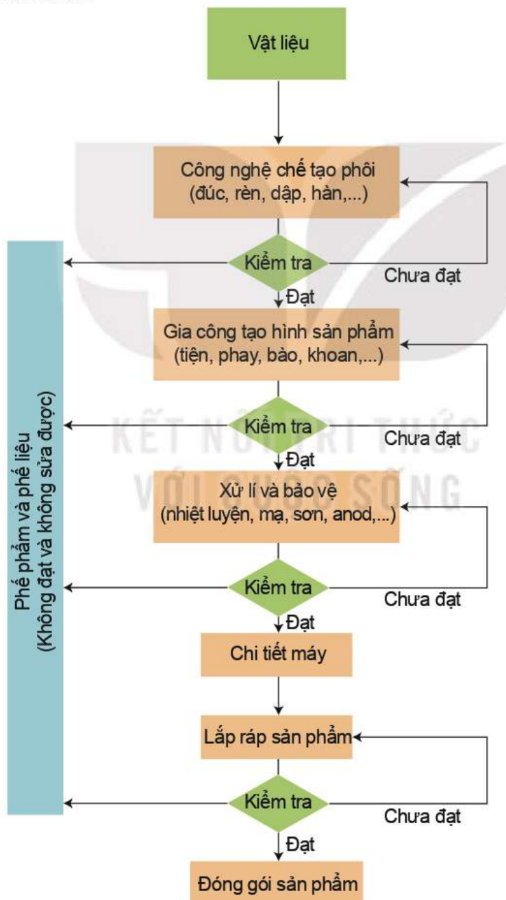
Hình 11.2. Quá trình sản xuất cơ khí
