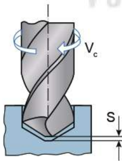
Hình 8.5. Thông số chế độ cắt khi khoan
