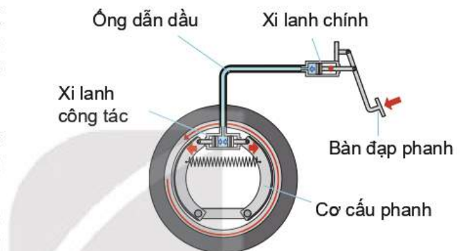
Hình 21.6. Hệ thống phanh
