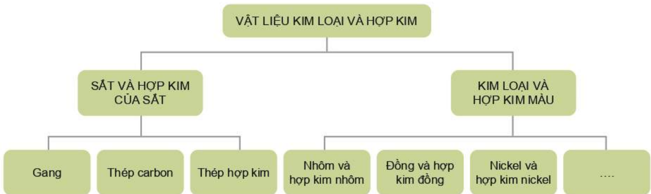
Hình 4.2. Phân loại kim loại và hợp kim
