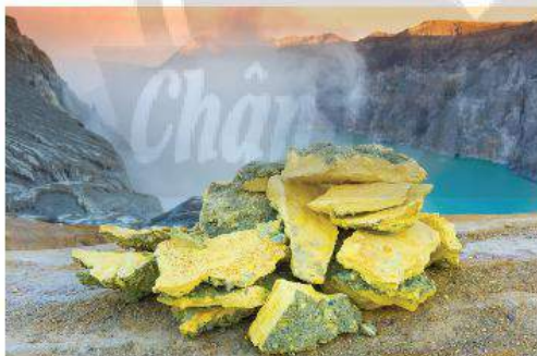
▲ Hình 6.1. Sulfur trong tự nhiên
