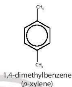
▲ Hình 14.2. Công thức cấu tạo và tên gọi một số hydrocarbon có vòng benzene
