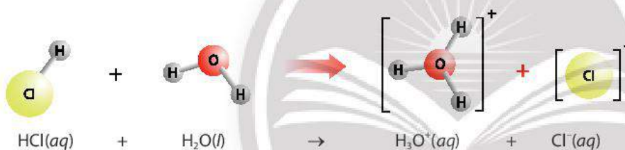
▲ Hình 2.4. Sơ đồ minh hoạ quá trình tương tác của \text{HCl} và nước trong dung dịch
