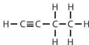
\text{CH}\equiv\text{C}-\text{CH}_2-\text{CH}_3 but-1-yne
