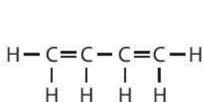
\text{CH}_2=\text{CH}-\text{CH}=\text{CH}_2 buta-1,3-diene
