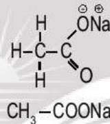
▲ Hình 8.3. Công thức cấu tạo một số hợp chất hữu cơ
