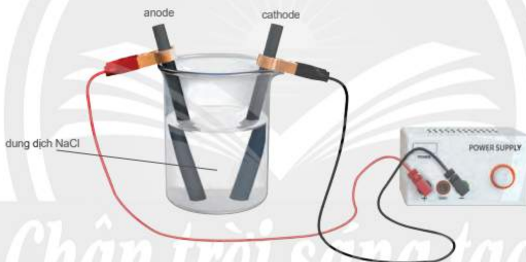
▲ Hình 13.2. Điện phân dung dịch NaCl
