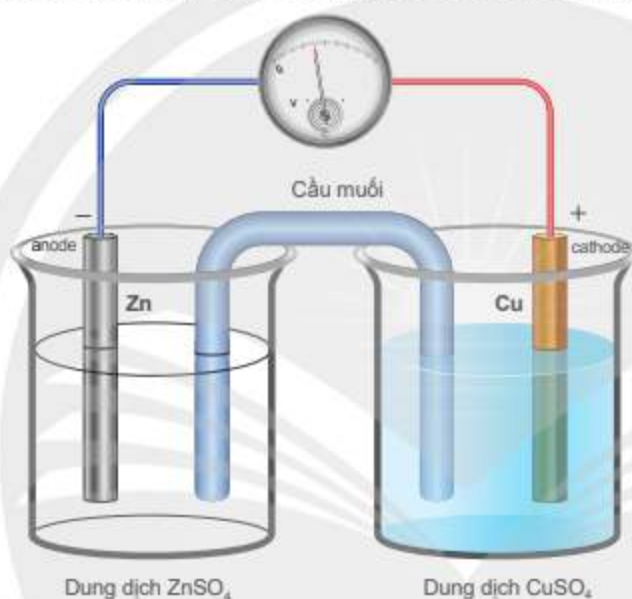
▲ Hình 12.1. Pin Galvani Zn-Cu
