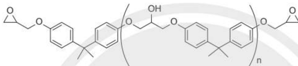
▲ Hình 11.2. Một loại keo dán epoxy
