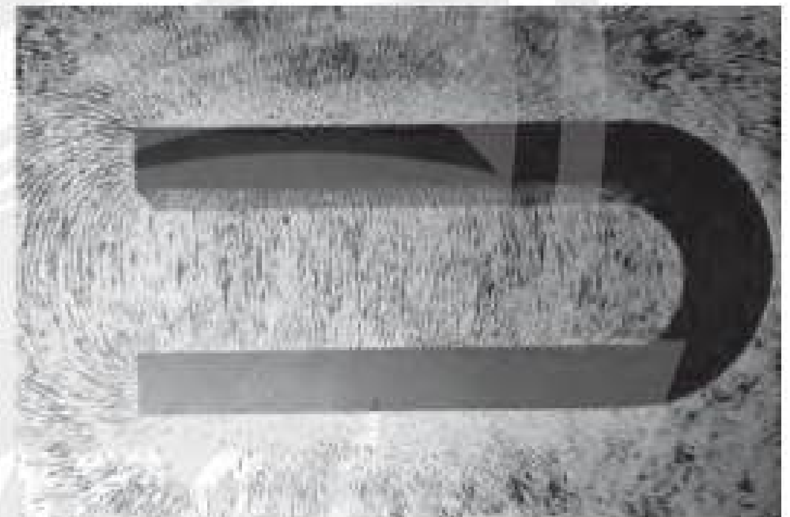
▲ Từ phổ của nam châm chữ U
