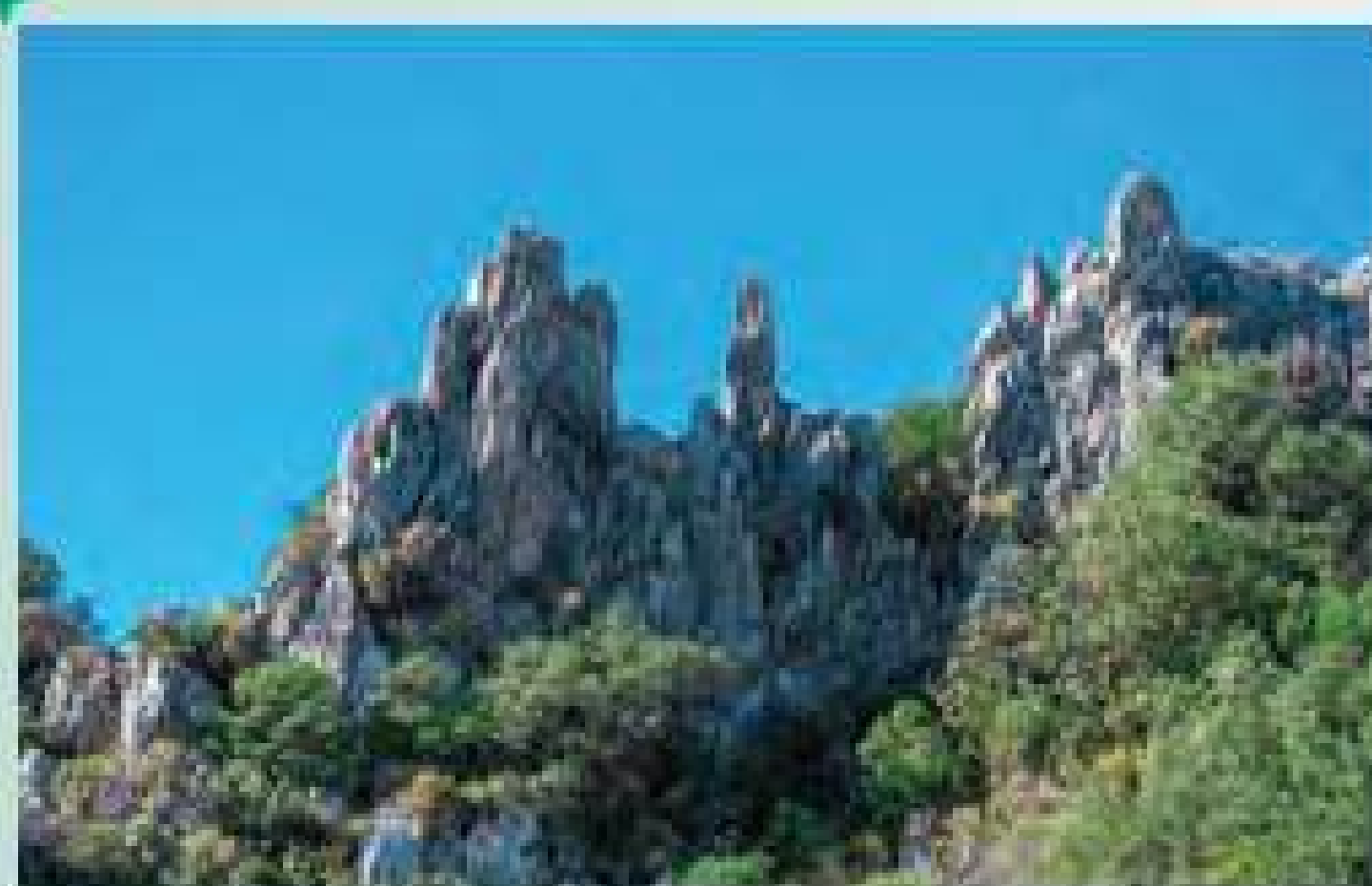
▲ Núi đá vôi
