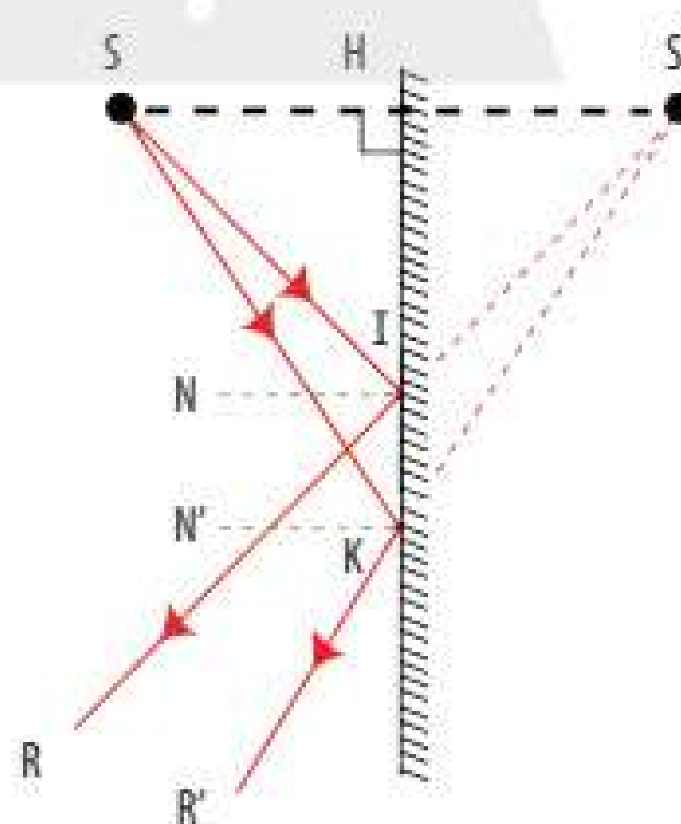
▲ Hình 17.3. Ảnh của điểm sáng S tạo bởi gương phẳng
