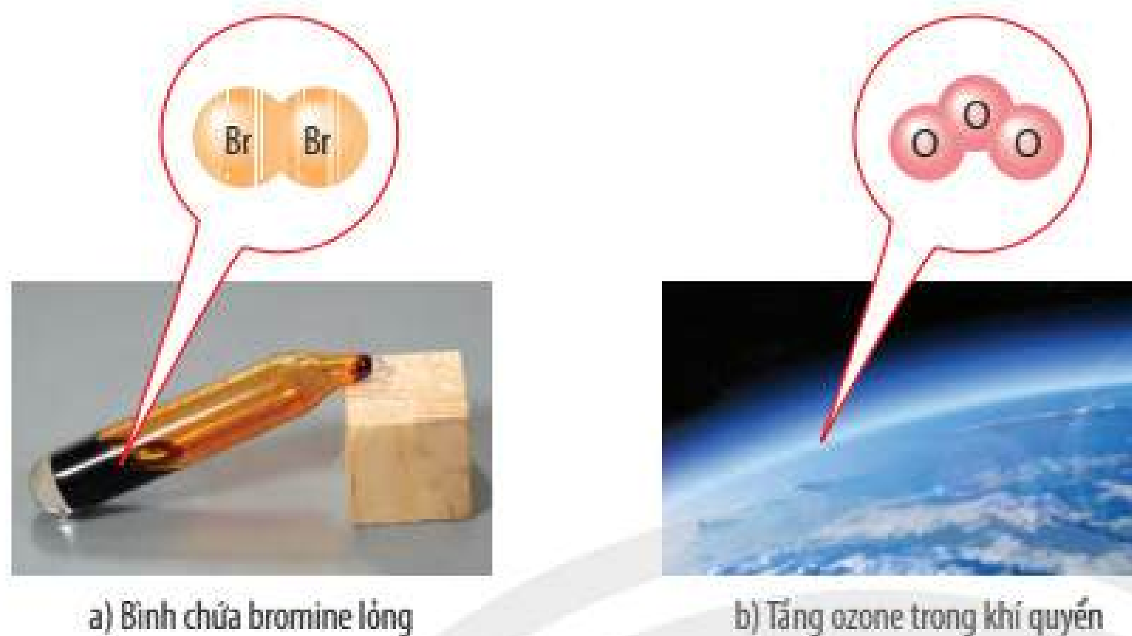
▲ Hình 5.6. Một số đơn chất và hình mô phỏng phân tử đơn chất
