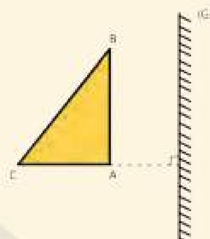
▲ Dựng ảnh của vật qua gương phẳng
