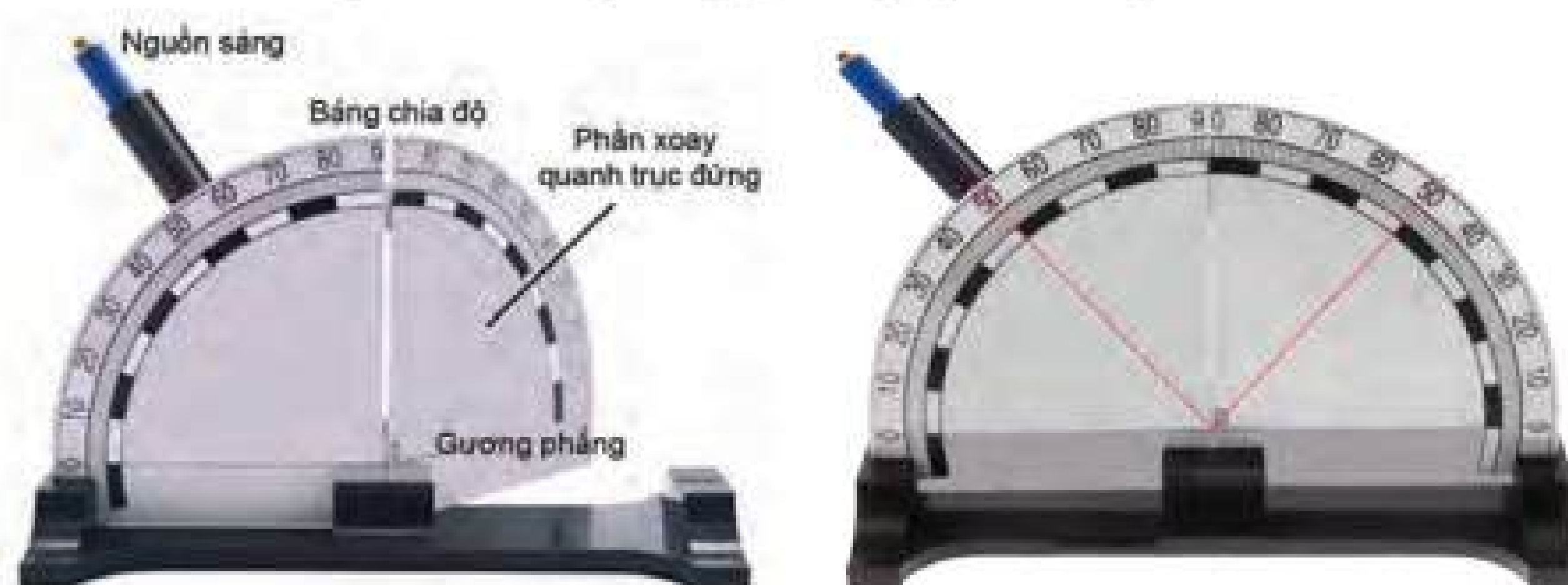
▲ Hình 16.3. a) Bố trí thí nghiệm; b) Quan sát tia sáng tới và tia sáng phản xạ khi nửa bên phải của bảng chia độ cùng mặt phẳng với nửa bên trái
