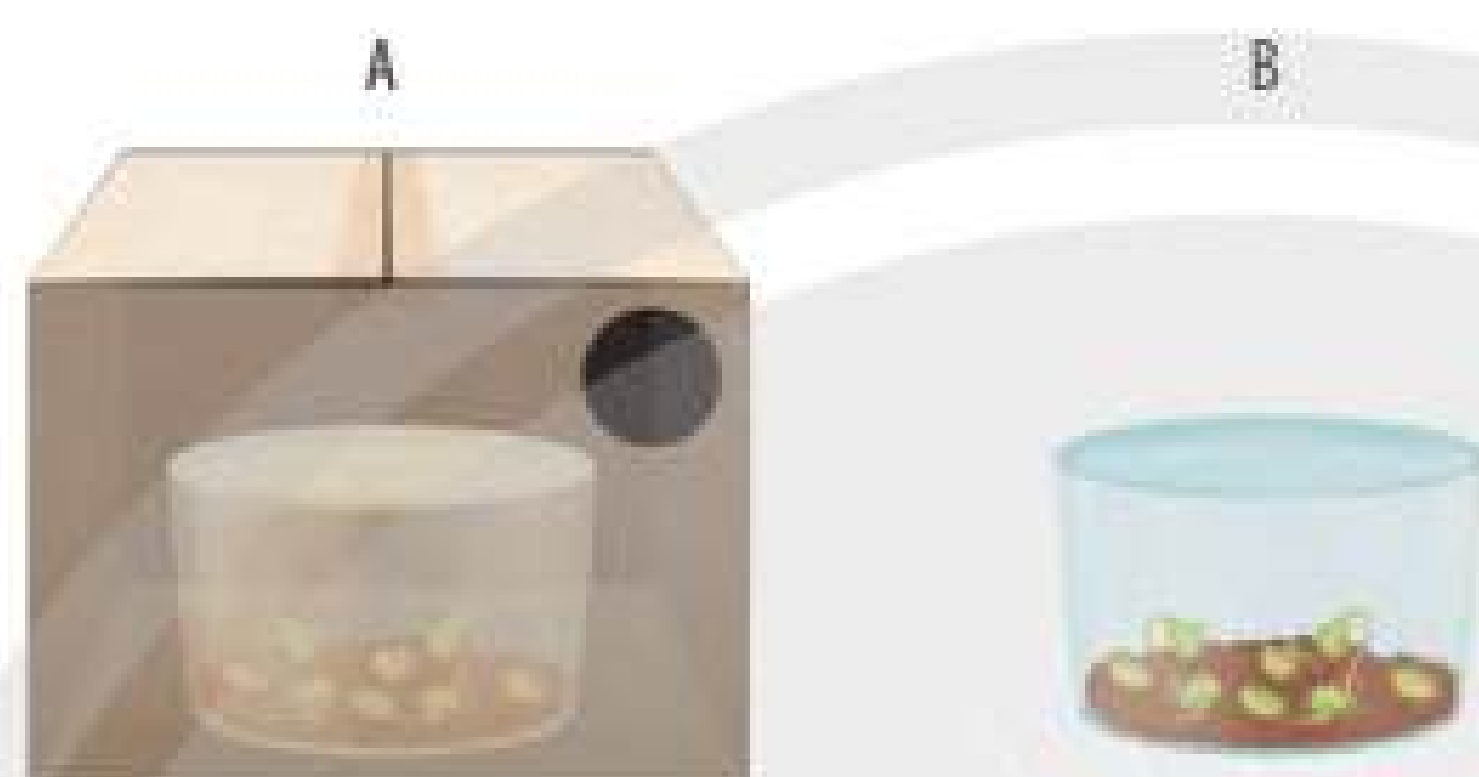
▲ Hình 32.5. Minh họa bước 2
