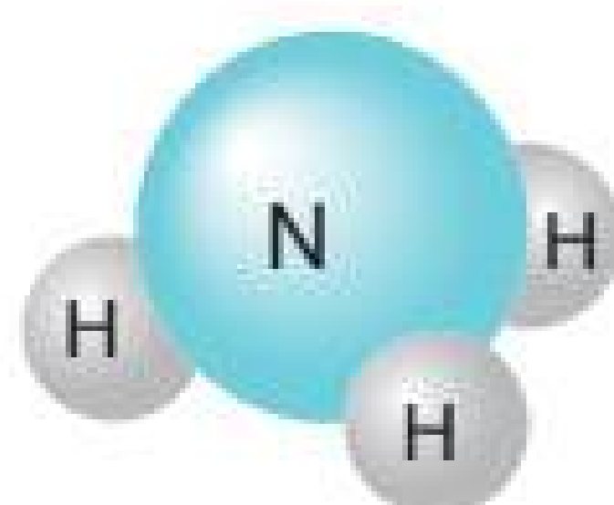
▲ Hình 5.4. Hình mô phỏng phân tử ammonia
