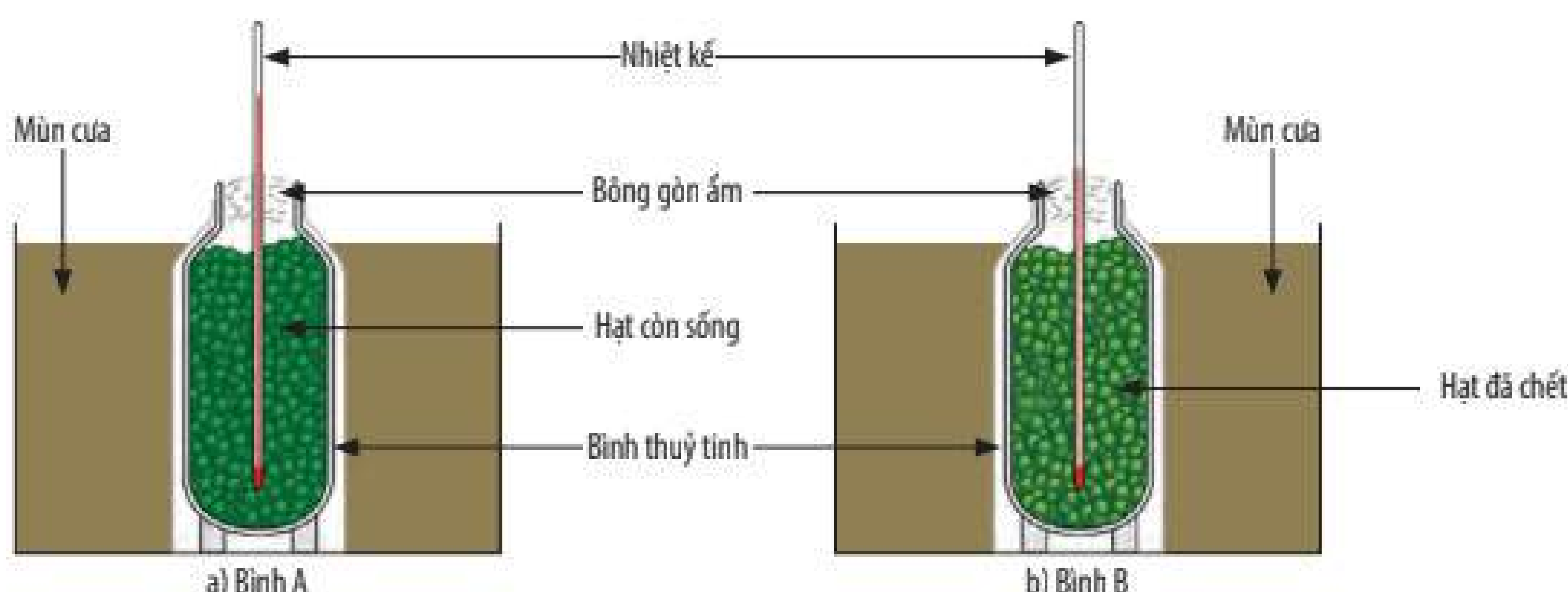
▲ Hình 26.1. Mô phỏng kết quả thí nghiệm
