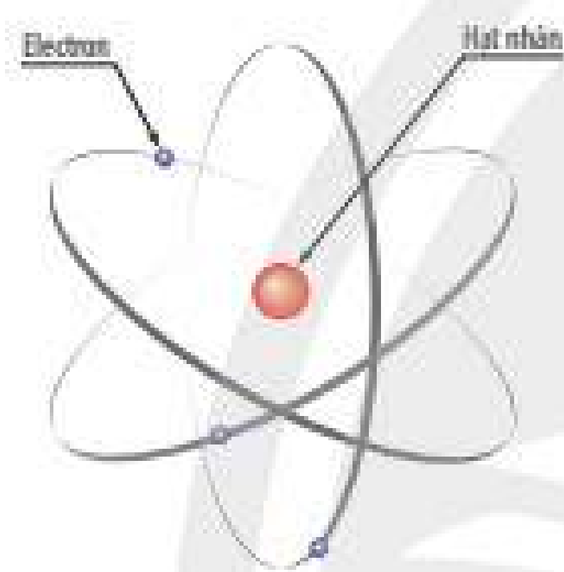
▲ Hình 2.4. Mô hình nguyên tử của Rutherford
