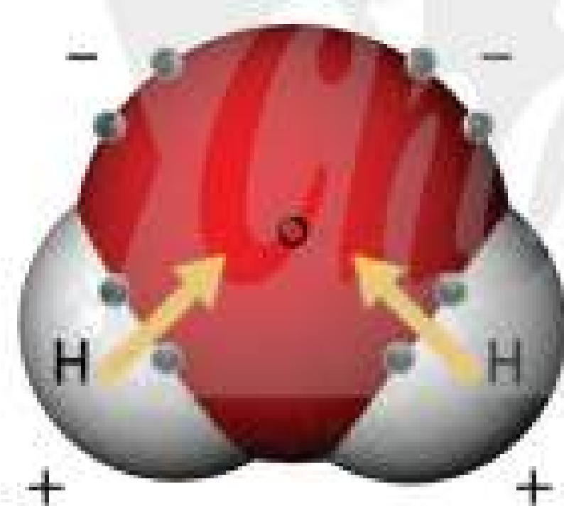
▲ Hình 28.1. Cấu trúc của phân tử nước
