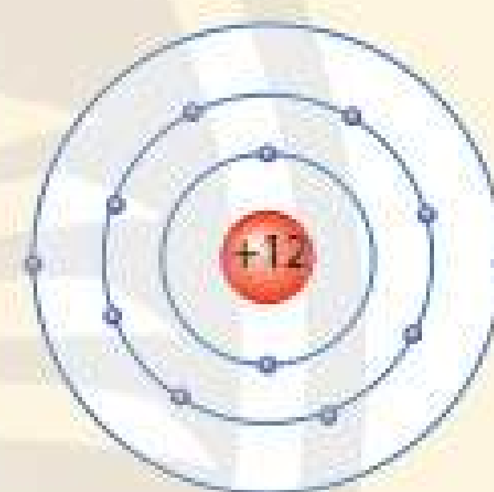
▲ Mô hình nguyên tử magnesium (Mg)
