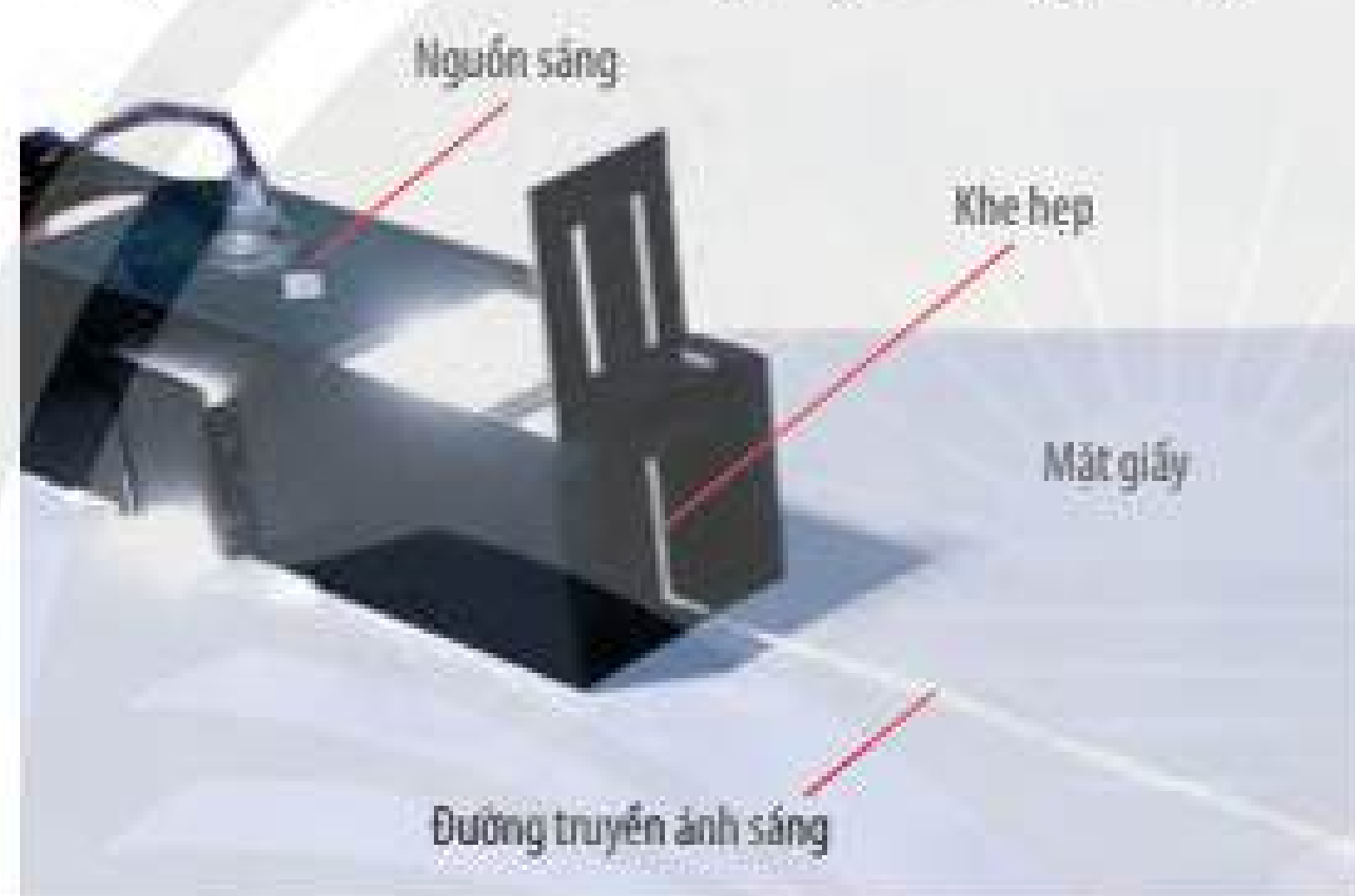
▲ Hình 15.3. Tạo chùm sáng hẹp song song
