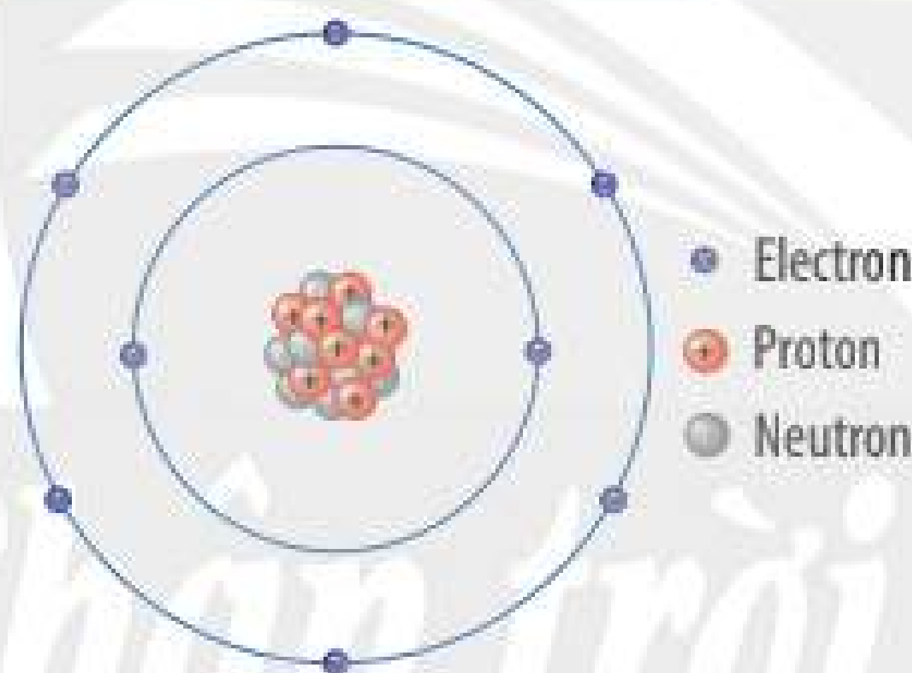
▲ Hình 2.6. Mô hình nguyên tử oxygen (O)
