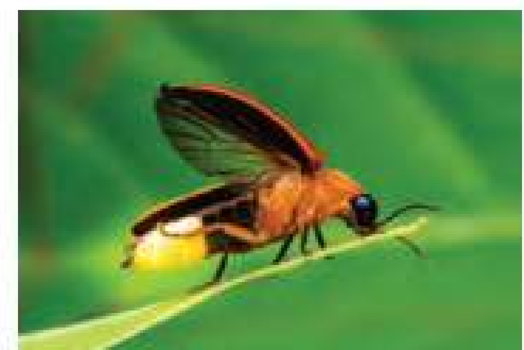
▲ Đom đóm đang phát sáng
