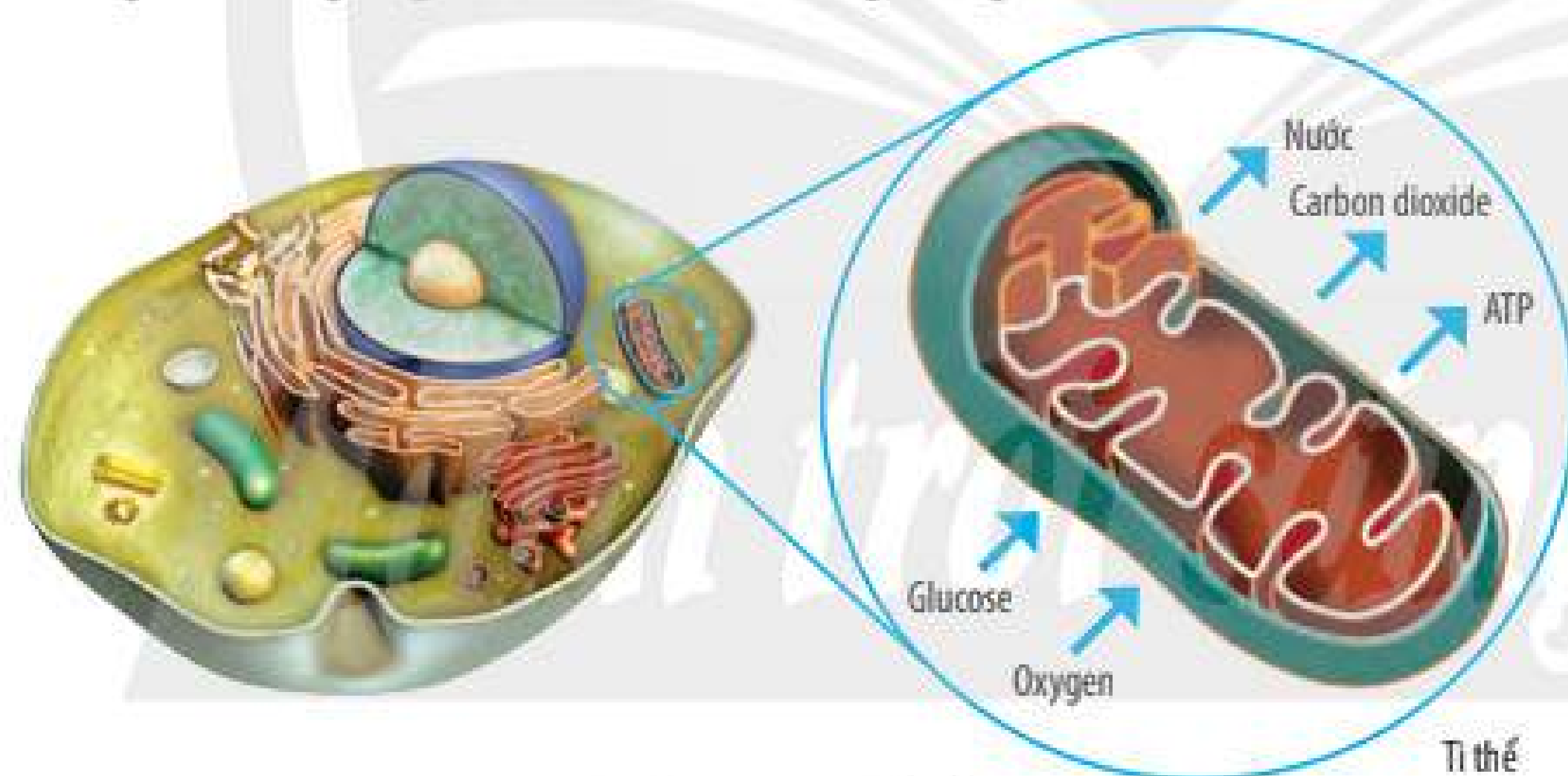
▲ Hình 25.1. Hô hấp tế bào
